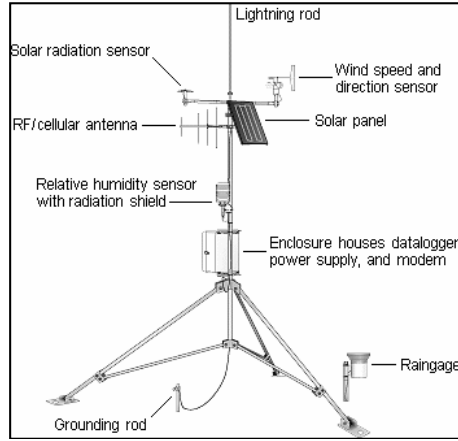
चित्र 1 स्वचालित मौसम स्टेशन चित्रण।
